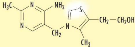
Thiamin
